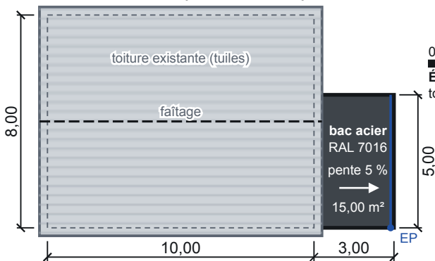
Plan de toiture (nord en haut)
